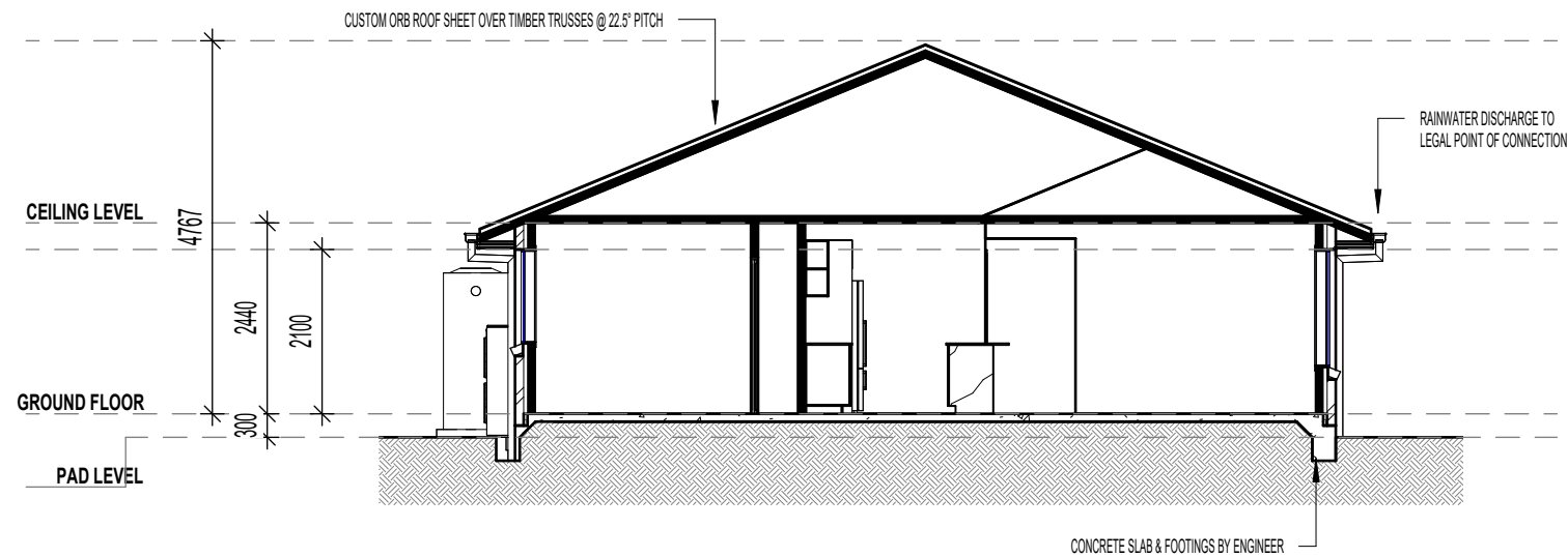
SECTION S2 1 : 100
