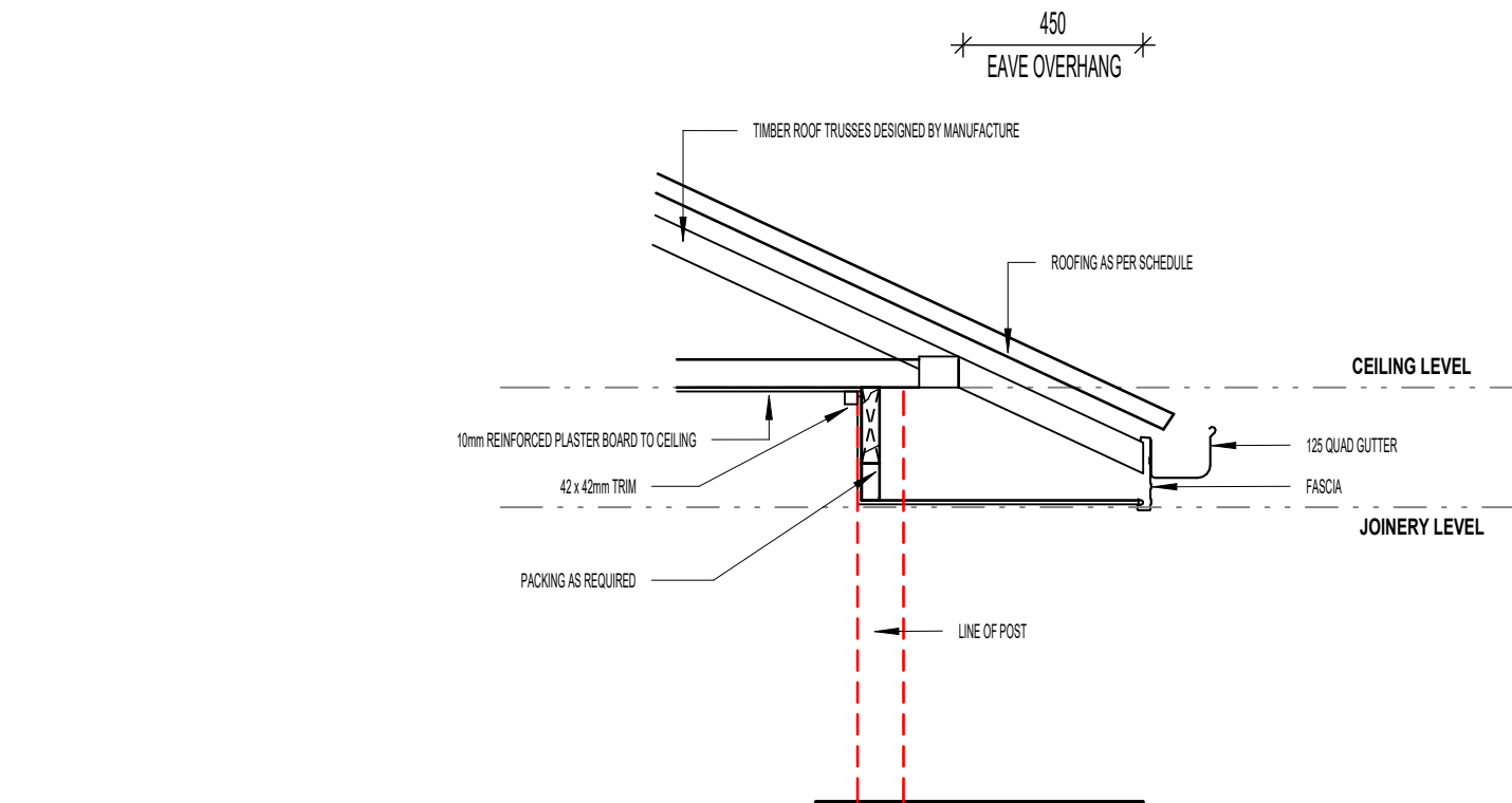
TYP. ALFRESCO EAVE DETAIL 1 : 20
