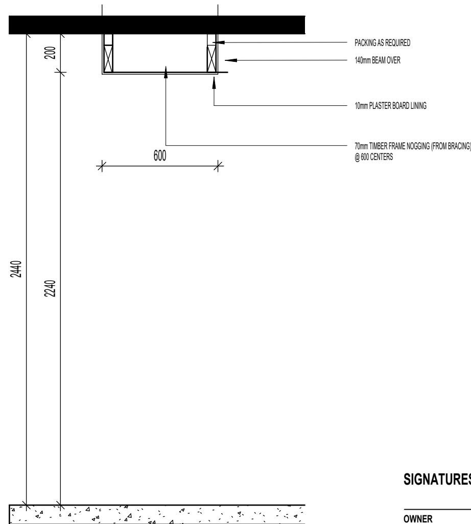
TYP. HALLWAY DETAIL 1 : 20
