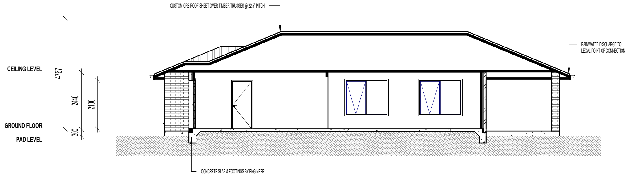
SECTION S1 1 : 100
